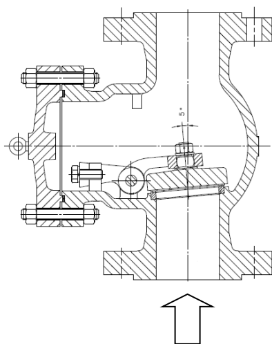
Montage Vertical ( fluide ascendant )
