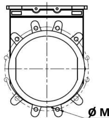
DN 450-500
