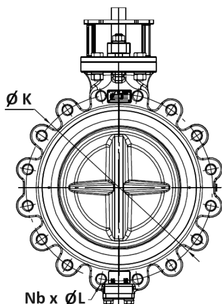
DN300-400
