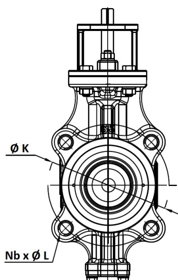
DN50
